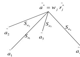
圖1 圖的範例
